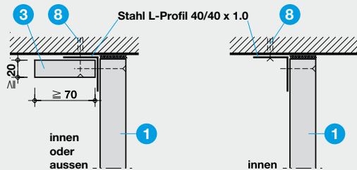
Detail F - Decken- Wandanschluss
