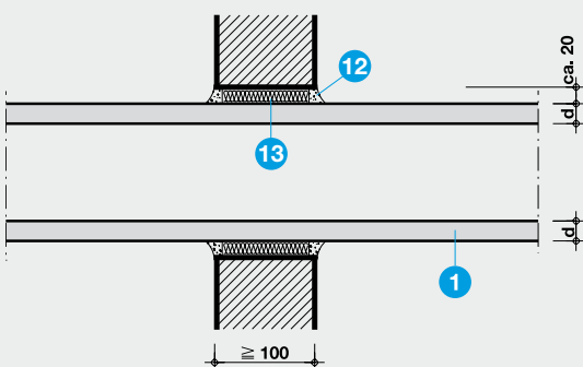
Detail D - Wanddurchführung
