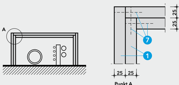
Detail E - Eckausbildung
