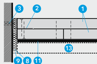
Schnitt A-A
