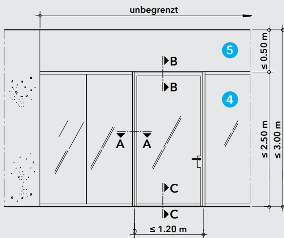
Ansicht - Einbau in Promat Ganzglaswand
