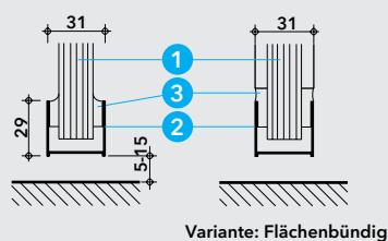
Detail C - Schnitt C-C
