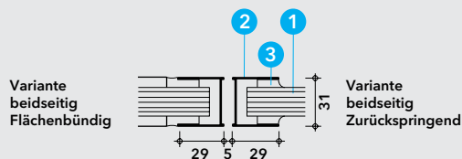
Detail A - Schnitt A-A
