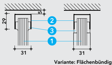
Detail B - Schnitt B-B
